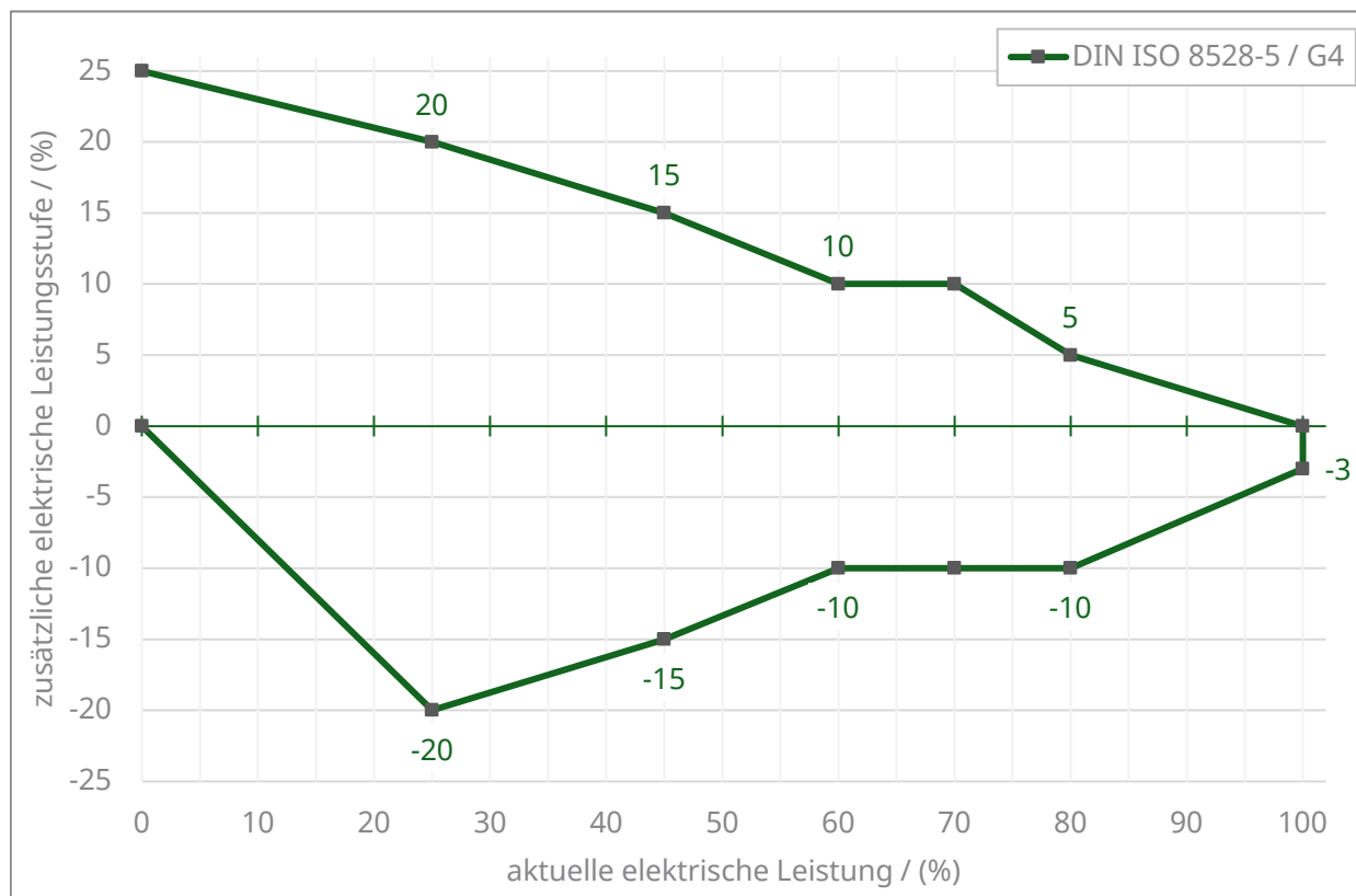
Lastaufschaltdiagramm
